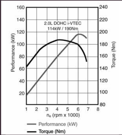
Effekt- och vridmomentskurva för 2,0 liters-motorn.
