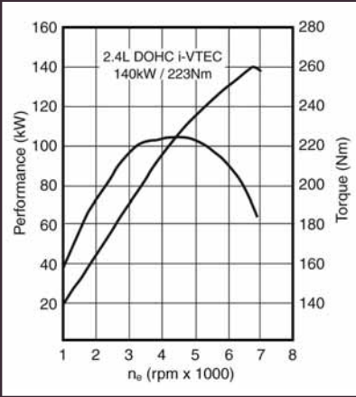
Effekt- och vridmomentskurva för 2,4 liters-motorn.
