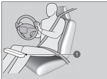
1 Krockkudde vid förarens knän, placering
