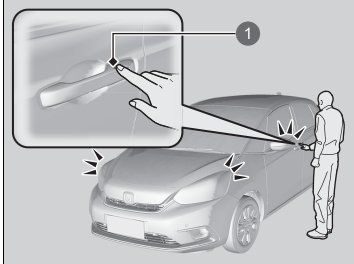
1 Dörrlässensor
