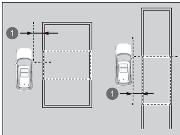
1 Ca 1 m
