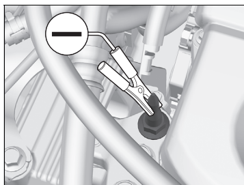
1 Hjälpbatteri
